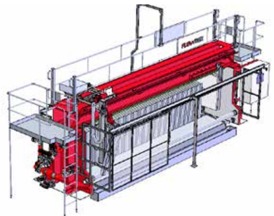
Flowrox proporciona modelos de filtro 3D precisos y un paquete de documentación completo, listo para incluir en el diseño de la planta.
