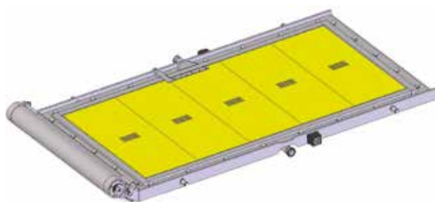
Фильтровальная пластина Flowrox W-16CR чашеобразная или плоская, правая или левая. Материал AISI 304, AISI 316, duplex 2205 или подобный.
