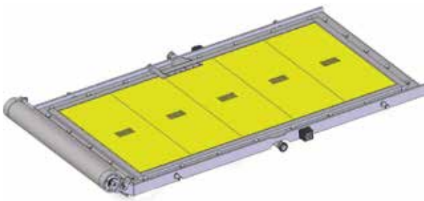
Placa filtrante W-16CR diseño ahuecado o plano, derecho o izquierdo. Material AISI 304, AISI 316, duplex 2205 o igual.
